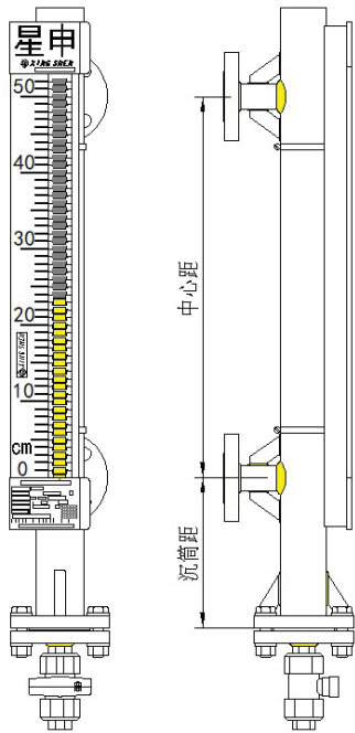
UHZ-517C16 结构简图
