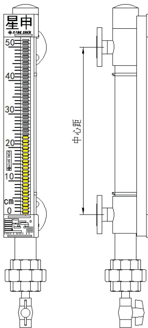
UHZ-517C17 结构简图
