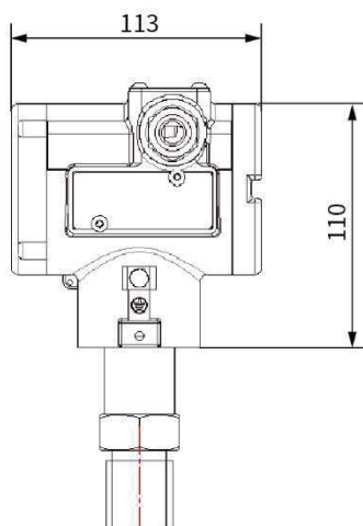
压力开关
