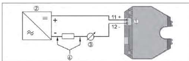
接线图（左）：
