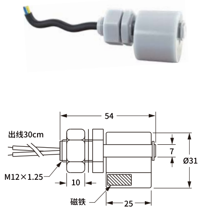
水平安装螺纹连接 UQK-501A526
