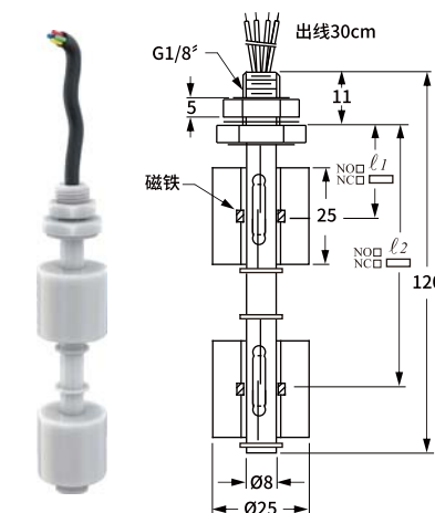
垂直安装两球螺纹连接 UQK-502A535
