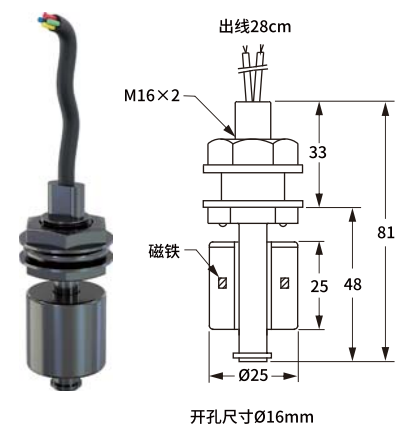
垂直安装螺纹连接(黑) UQK-502A535
