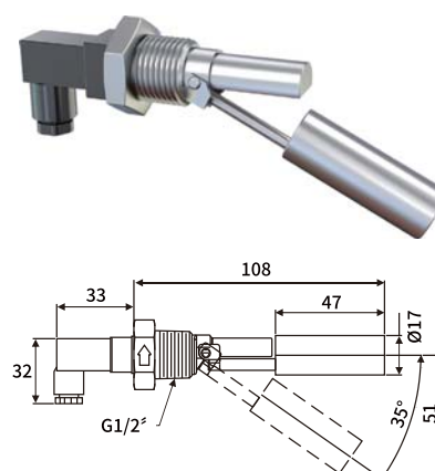
水平安装螺纹连接(弯头接线) UQK-501A526
