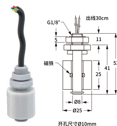
垂直安装螺纹连接 UQK-502A535
