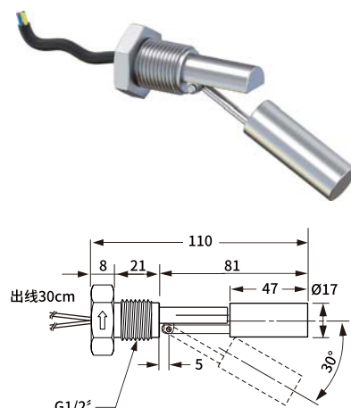
水平安装螺纹连接(短浮子) UQK-501A526
