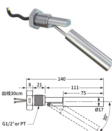
水平安装螺纹连接(长浮子) UQK-501A526
