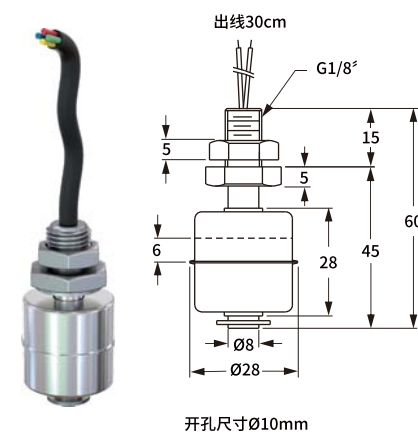
垂直安装螺纹连接 UQK-502A525
