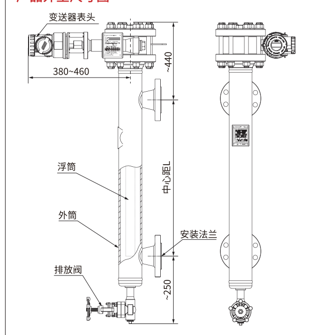
产品外型尺寸图
