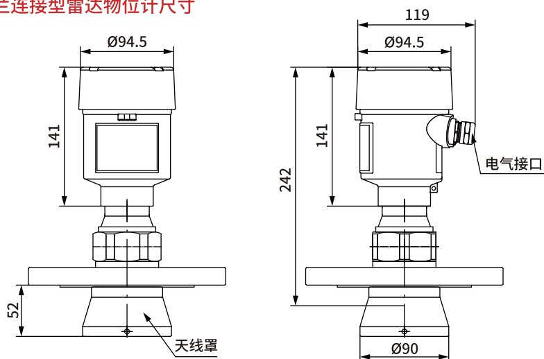
法兰连接型雷达物位计尺寸
