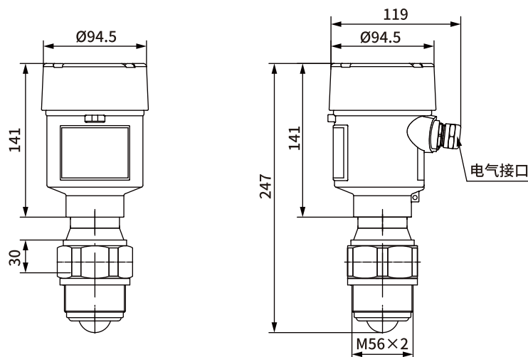
螺纹连接型雷达物位计尺寸
