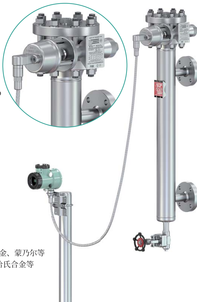
产品安装示意图
