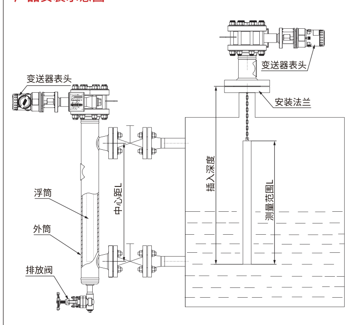
产品安装示意图
