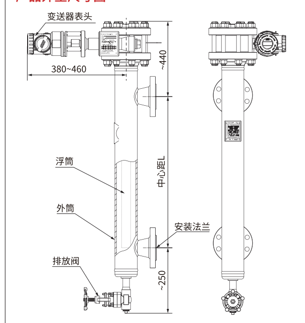
产品外型尺寸图
