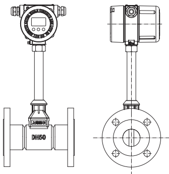
SM2系列涡街流量计结构图-法兰不带散热片
