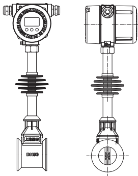
SM2系列温压补偿涡街流量计结构图-法兰式
