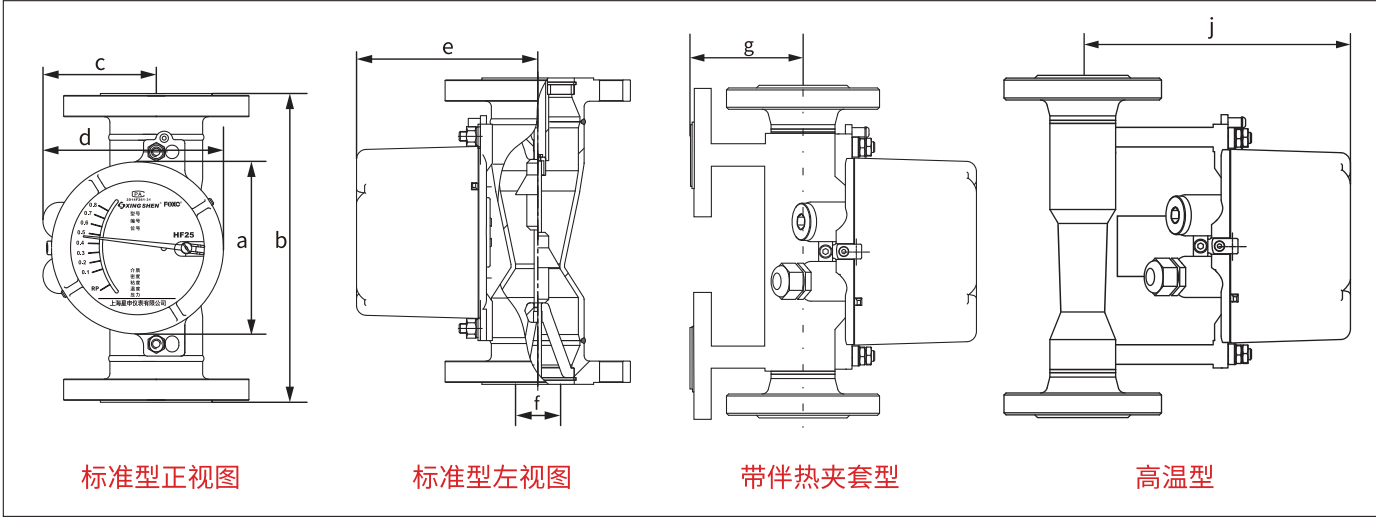
产品外形结构尺寸简图:
