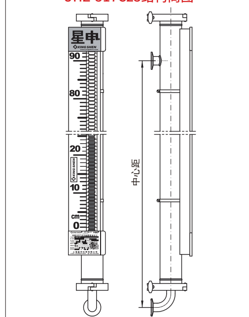
UHZ-517C23结构简图
